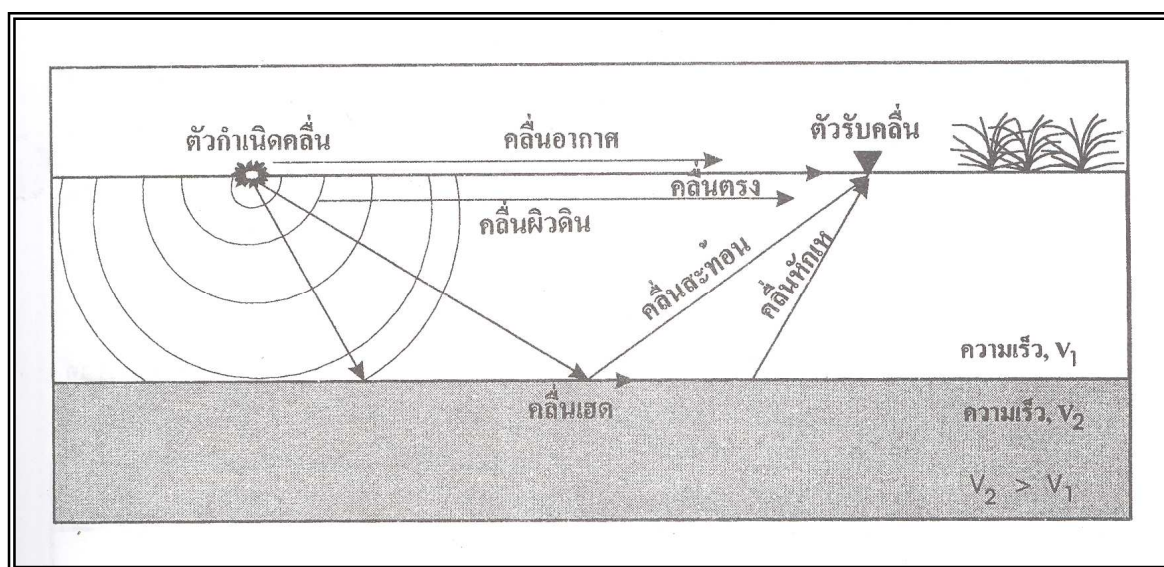
รูปที่ 2.1 แสดงลักษณะภาพจำลองโดยการสำรวจ ธรณีวิทยาใต้พื้นผิวด้วยคลื่นไหวสะเทือนแบบหักเห (Seismic Refraction Exploration) (4)
