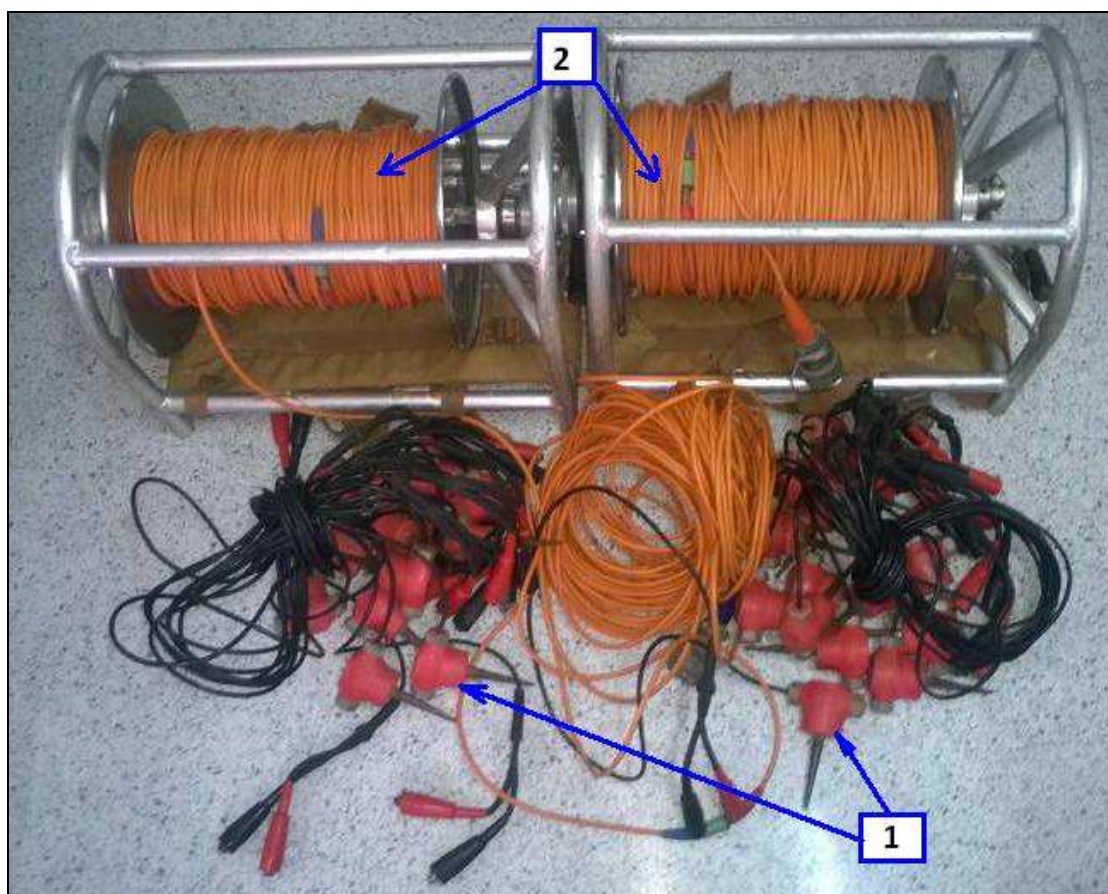
รูปที่ 3.2 แสดงลักษณะรูปร่างของ จีโอโฟน และสายนำสัญญาณ
